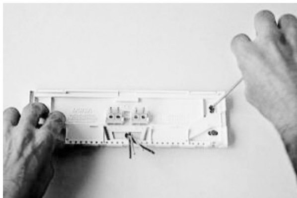
Visser la plaque de fixation
